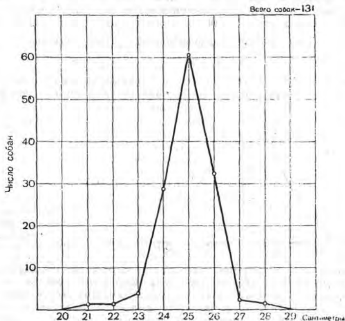
Рис. 8. Графическое изображение воображаемого ряда изменчивости (ряд II) для сравнения с рис. 5 (ряд I). Квадратическое уклонение ряда I=1,38, ряда II=0,94. Пределы колеблемости одинаковы (Ориг.).
